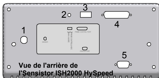
Fig 3-2. Ports et connexions de l'Sensistor ISH2000 HySpeed.
