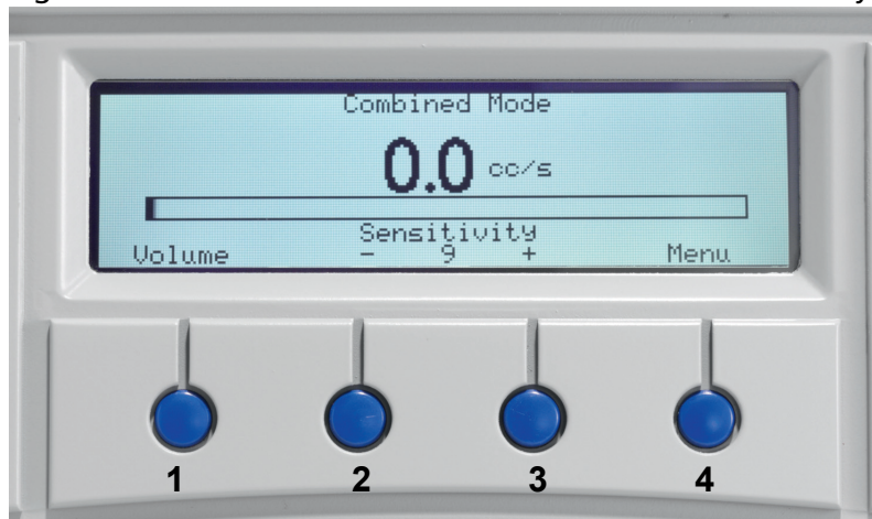
Fig 8-1. Commandes et indicateurs de l'Sensistor ISH2000 HySpeed.
