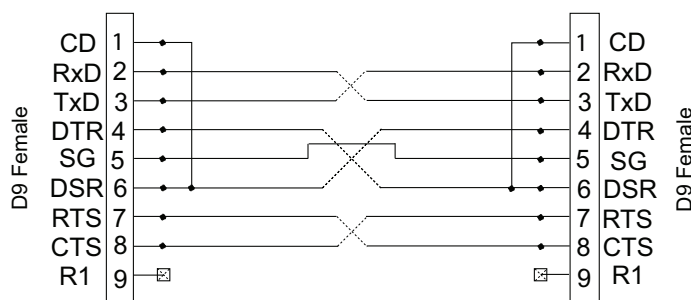
Bild 8-5. Kopplingsschema för nullmodemkabel D9
